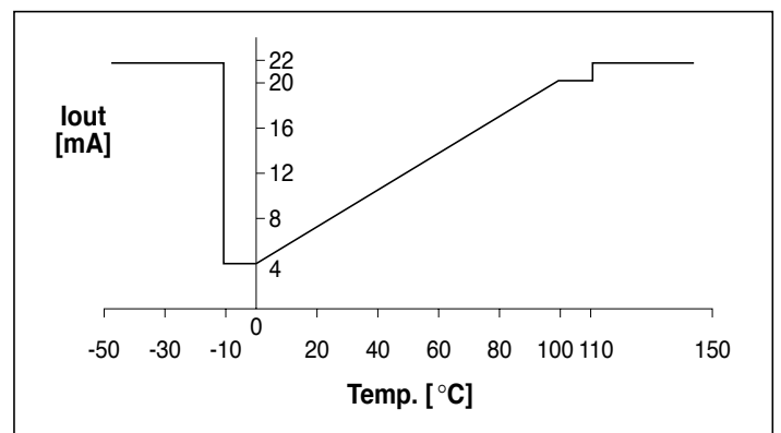
Fig. 1 Range 0...100°C, corrente di uscita in funzione della temperatura.
